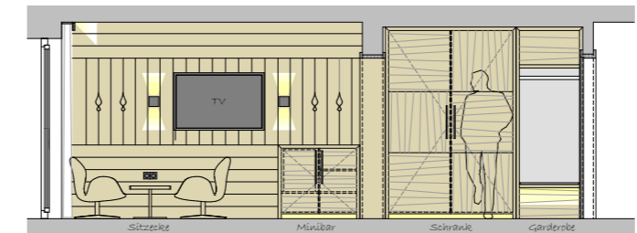
Wandansicht Aufenthaltsbereich
